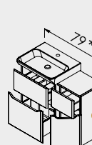
50x70x40cm PIXI 50
