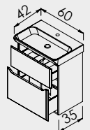
60x70x42cm PIXI 60
